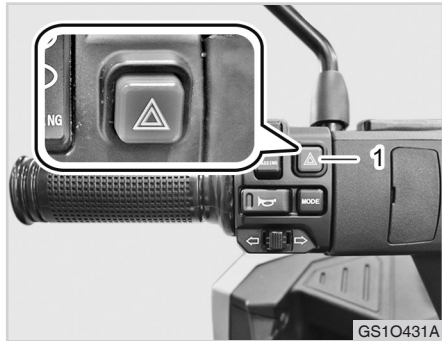
(1) 비상등 버튼
