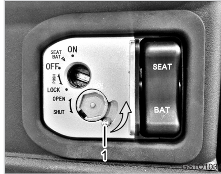
(1) 잠금 레버
